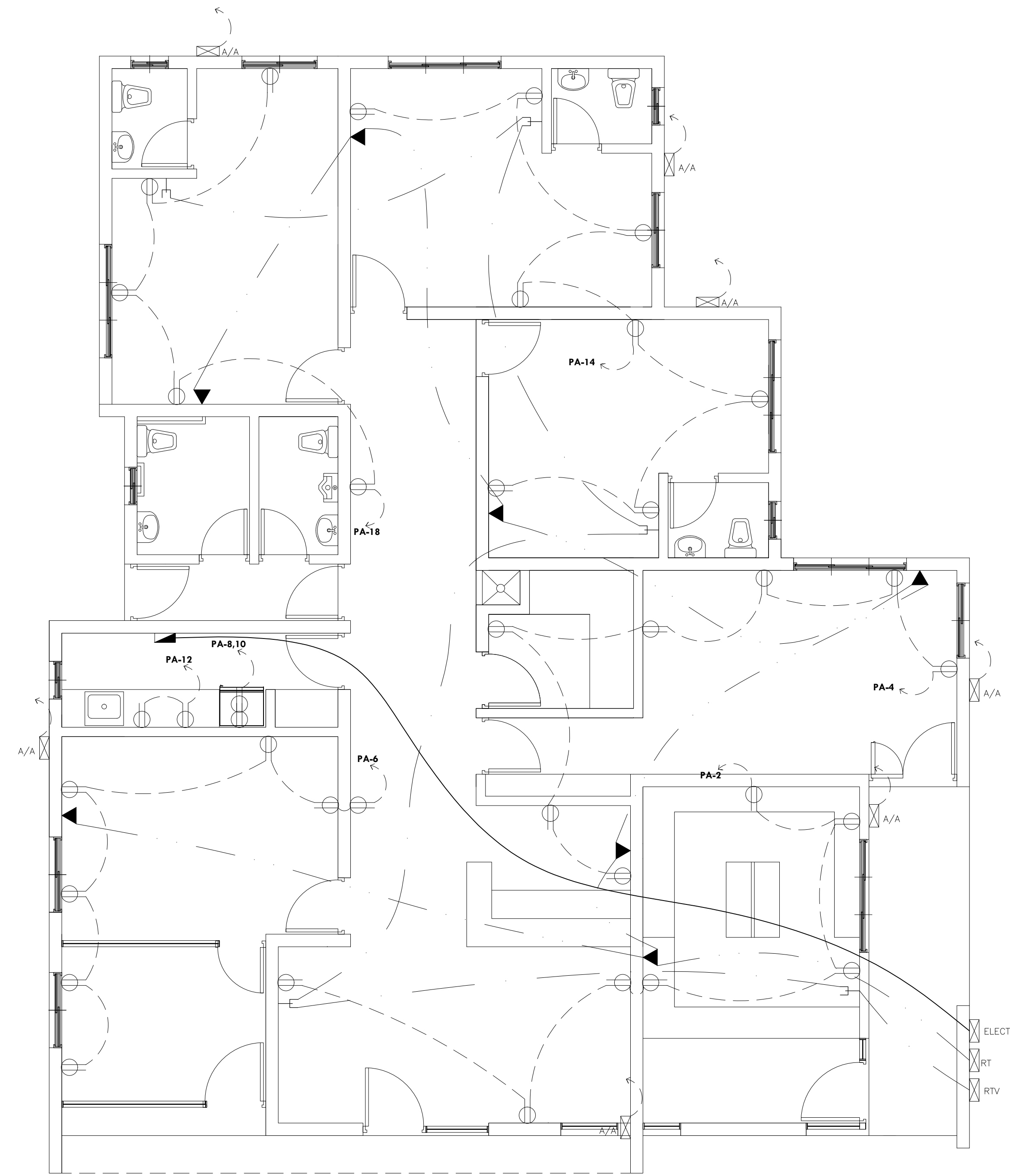
DISPENSARIO MEDICO MAMACHEN PLANTA ELECTRICA TOMACORRIENTES [ESC.: 1:50]
