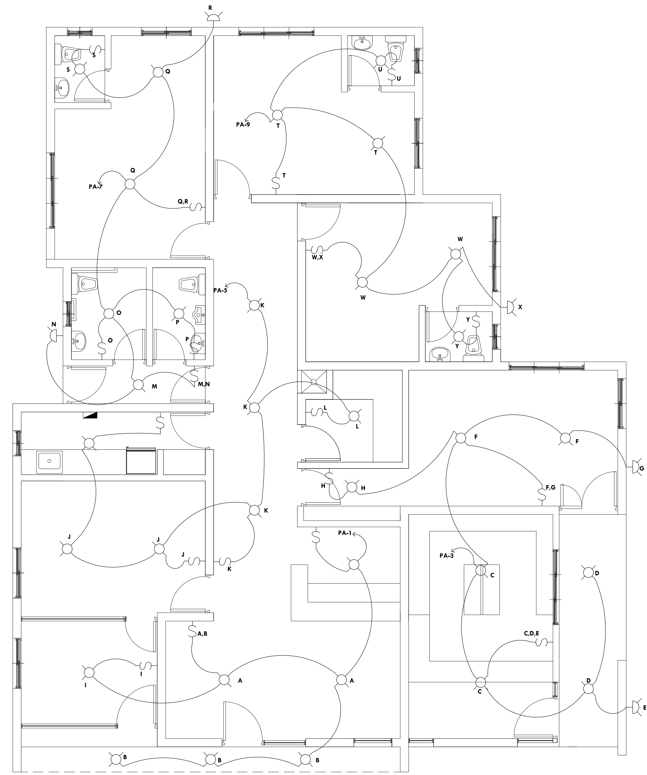
DISPENSARIO MEDICO MAMACHEN PLANTA ELECTRICA LUMINARIAS [ESC.: 1:50]
