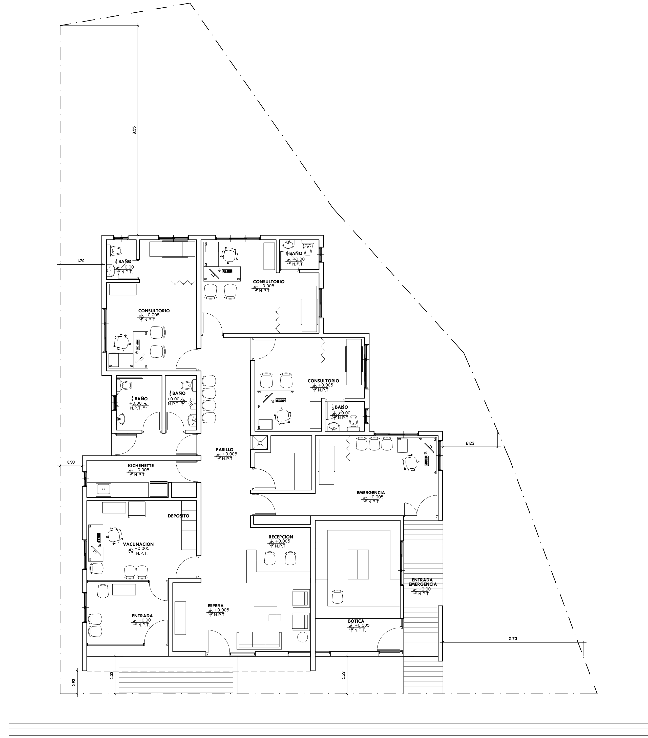
DISPENSARIO MEDICO MAMACHEN PLANTA UBICACION EN EL SOLAR [ESC.: 1:75]
