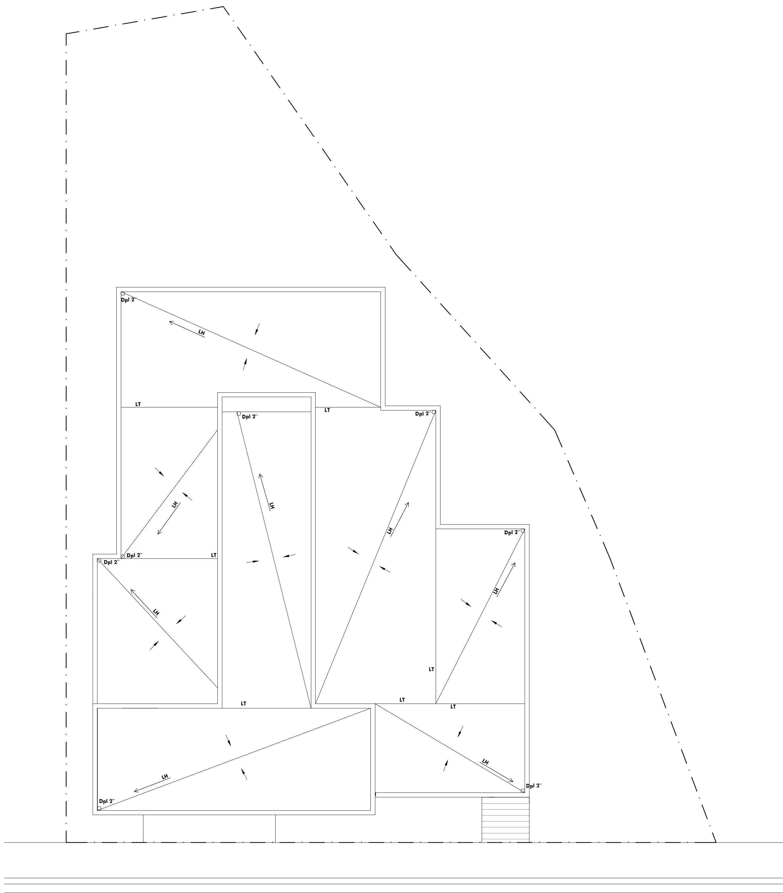
DISPENSARIO MEDICO MAMACHEN PLANTA DE TECHO [ESC.: 1:75]
